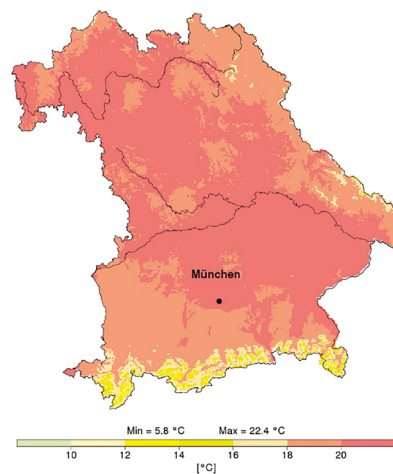
Lufttemperatur August 2018
