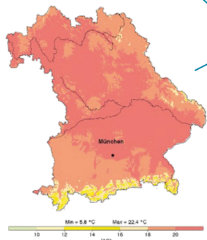
Lufttemperatur August 2018
